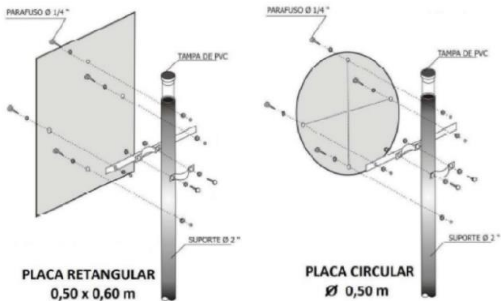
Figura 2 - Disposição dos Furos e Instalação das Placas de Sinalização.
