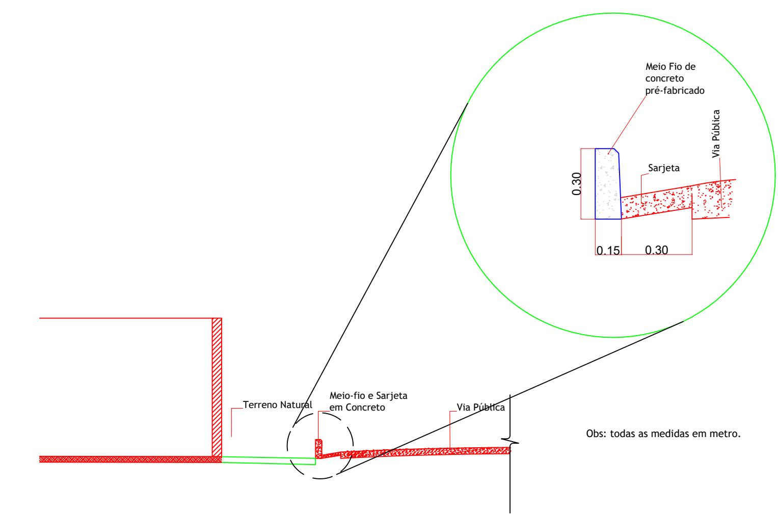
DETALHE DRENAGEM SUPERFICIAL S/ ESCALA
