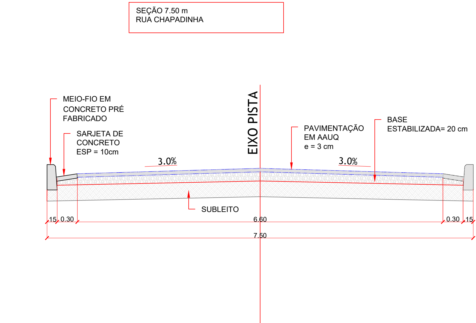
Seção Transversal - Seção 7.50 m SEM ESCALA
