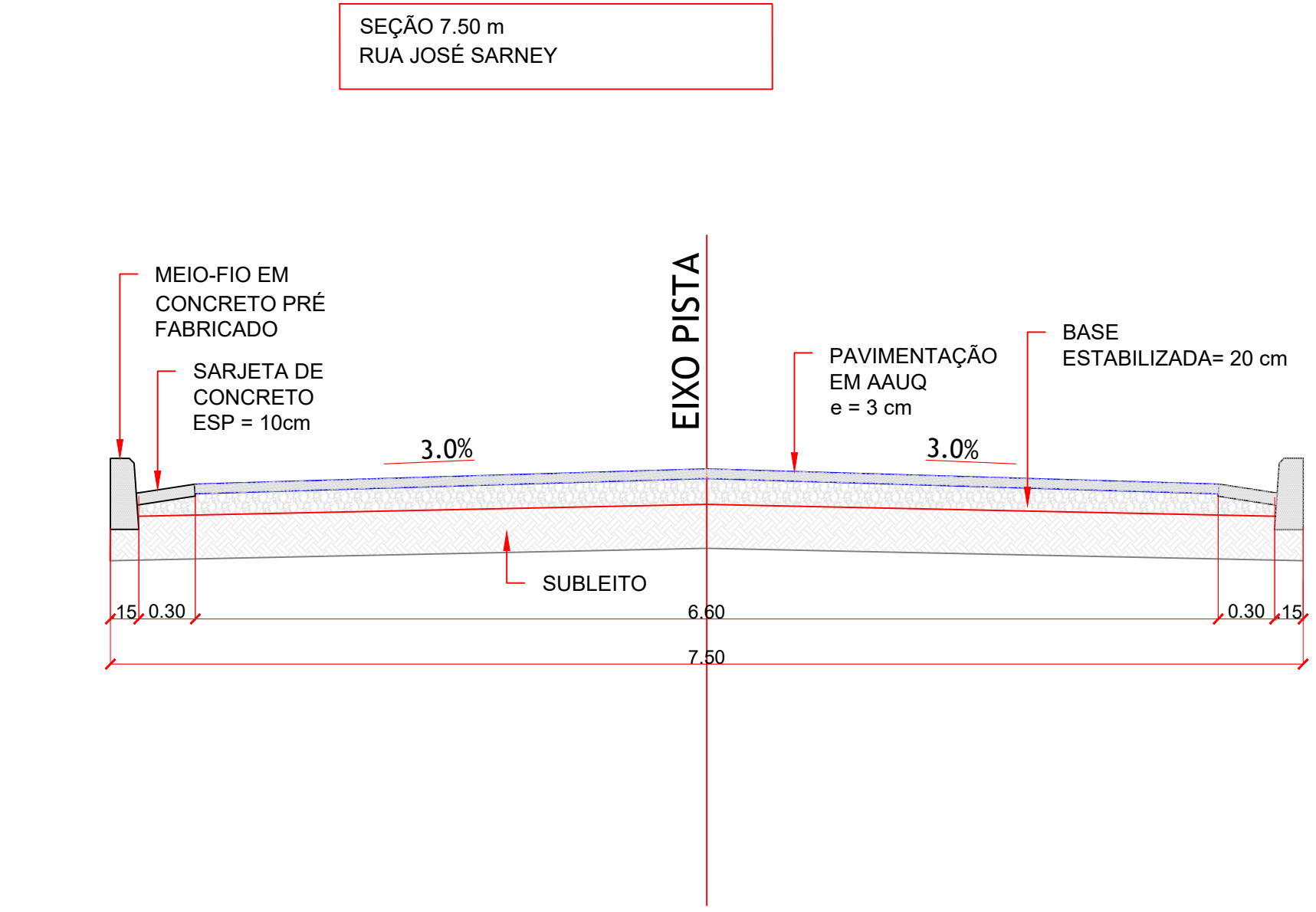
Seção Transversal - Seção 7.50 m SEM ESCALA
